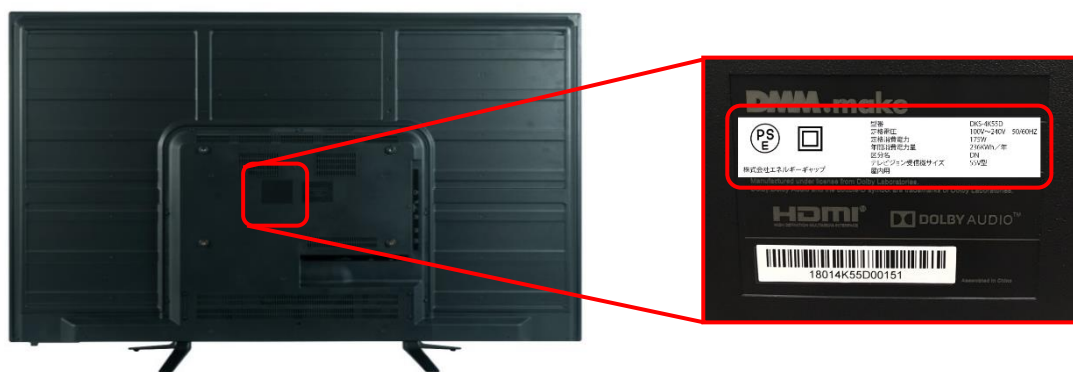
背面図
